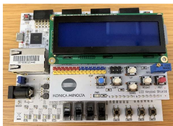
Artix-7 35T Arty FPGA 評価キット LCDシールドボード (LCD Keypad Shield for Arduino互換品)
